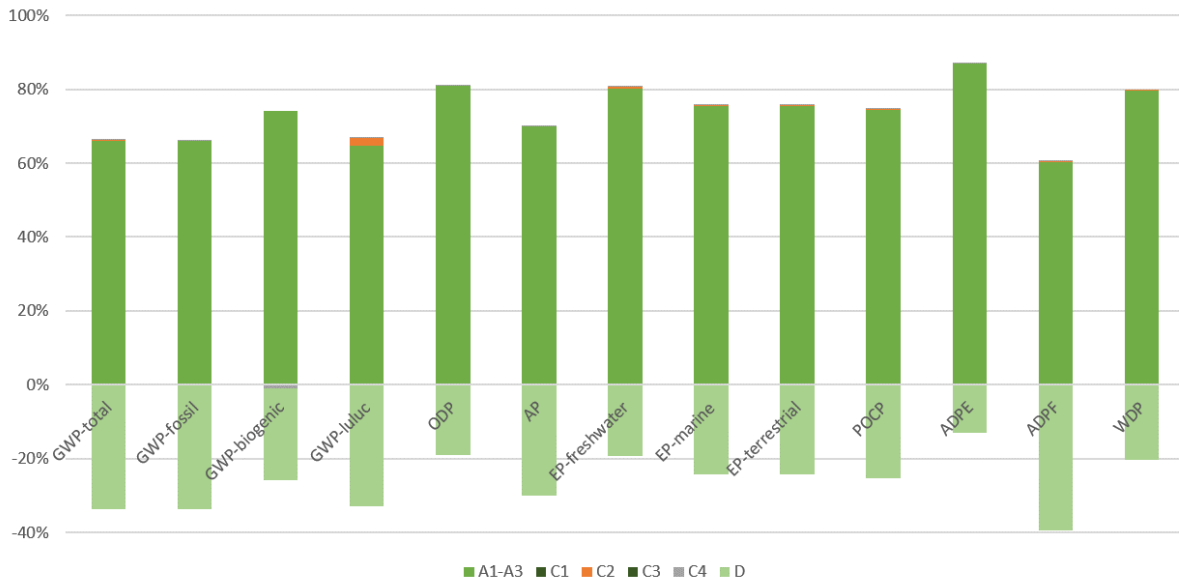
Relative Beiträge der verschiedenen Lebenszyklusphasen der Aluminium-Strangpressbolzen
